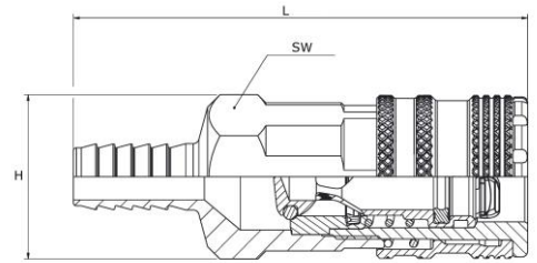
Schlauchanschluss
