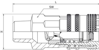
Außengewinde
