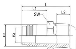
Nippel Außengewinde
