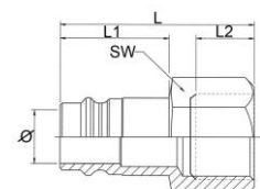
Nippel Innengewinde
